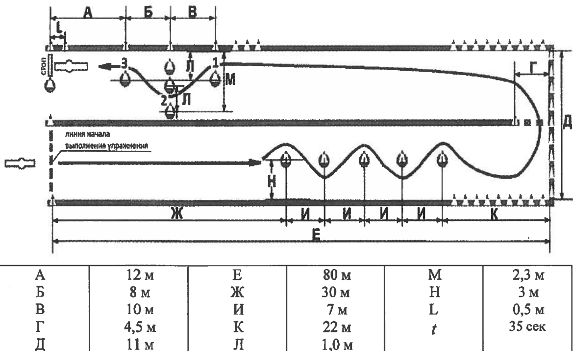
Рисунок 3. Схема и размеры элемента упражнения № 1 – «Скоростное маневрирование»
