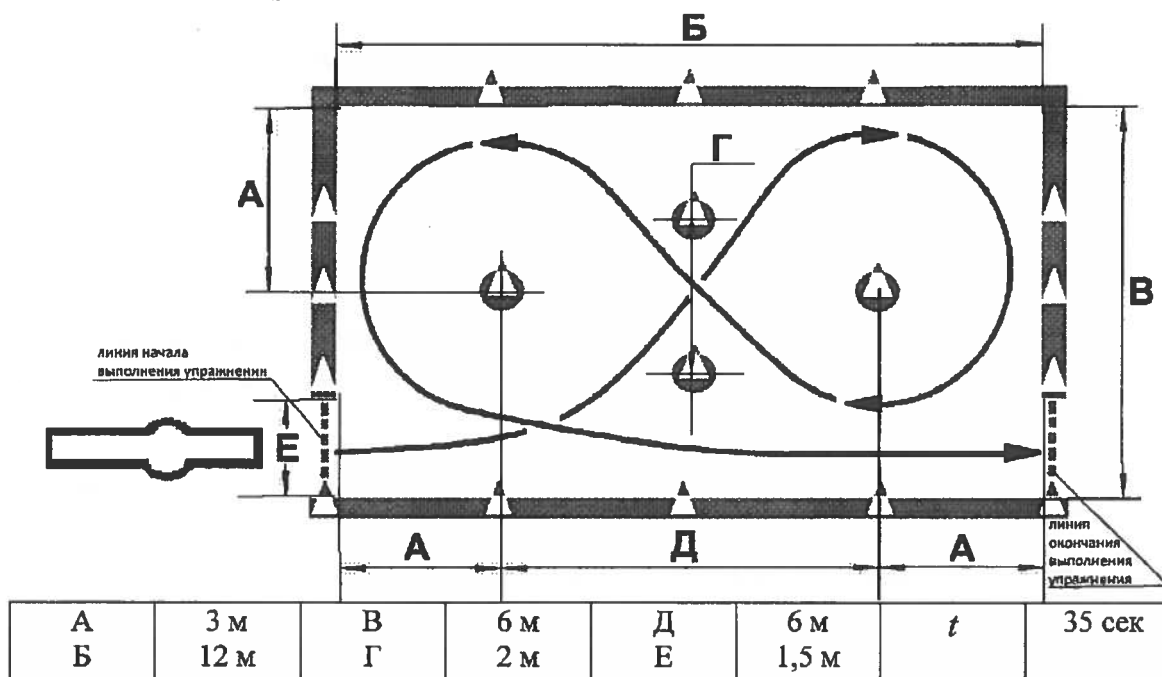
Рисунок 1. Схема и размеры элемента упражнения № 1 - «Габаритная восьмерка»
